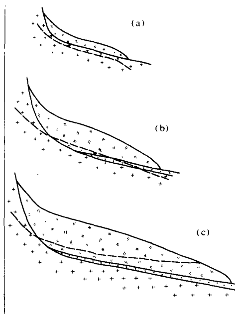
图2 我国亚极地型冰川的三种模式
