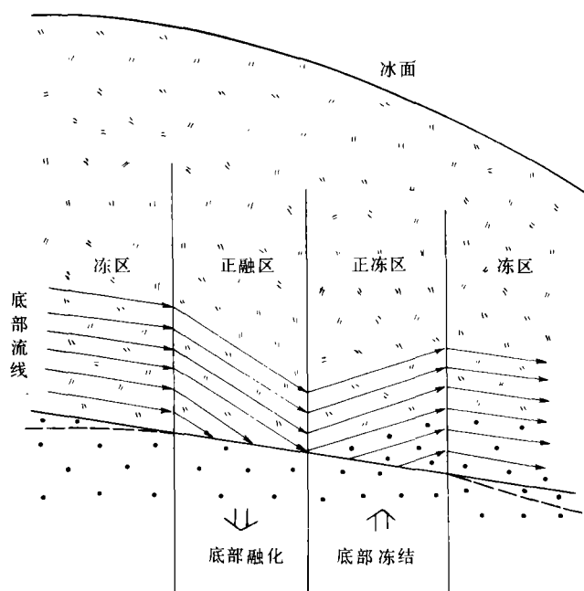
图 3 冰下融区的融化-冻结过程示意图
