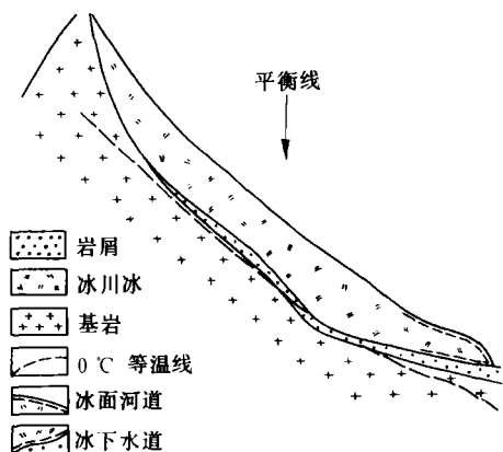
图 1 1号冰川东支冰床特征示意图
