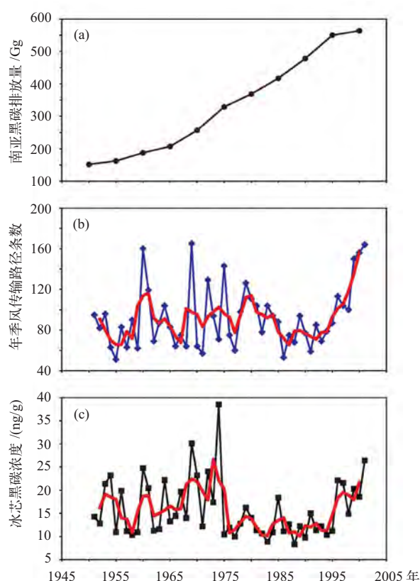
图 6 1950—2000 年南亚地区的黑碳排放变化 (a) [26] , 1951—2001 年逐年印度夏季风输送的气团轨迹条数 (b), 东绒布冰芯记录的黑碳浓度 (c) (红色曲线为滑动平均)
