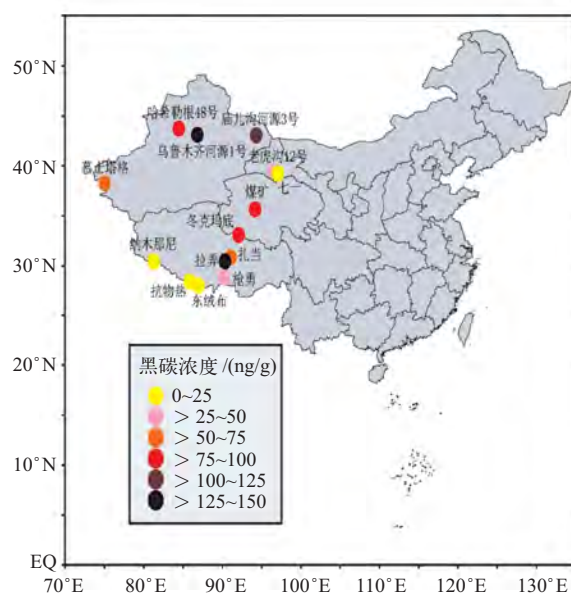
图2 中国西部冰川雪样黑碳浓度分布图
