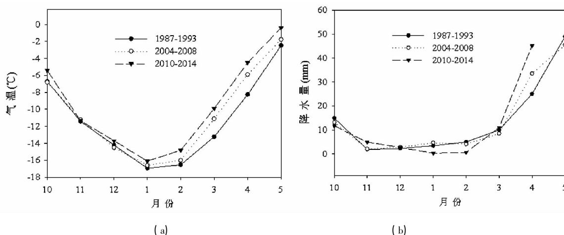
图3 空冰斗冬、春季气温与降水的变化趋势
